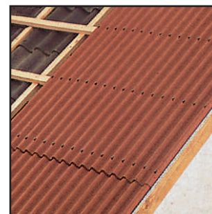
Schéma postupu laťování při pokrývání staré střechy
