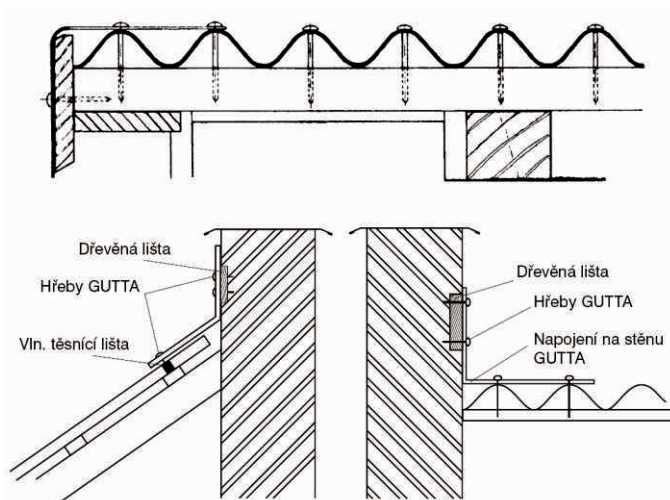
Schéma napojení na stěnu - boční
