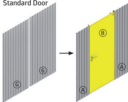
Standard Door
