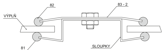
Střešní sloupky
