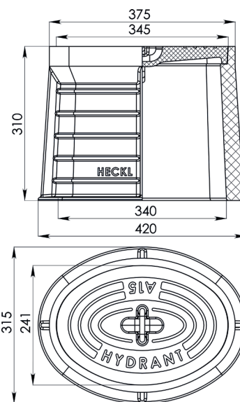
Hydrantový poklop
